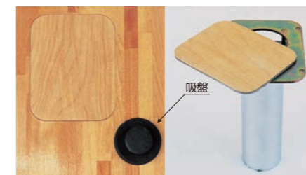
VT-6258 バレー・テニスポスト用床金具 <フローリング貼>
