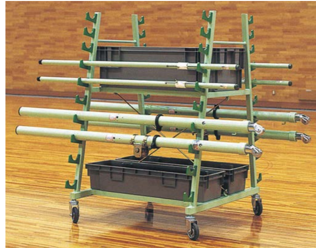
GF-3133 器具収納車<20本掛>
